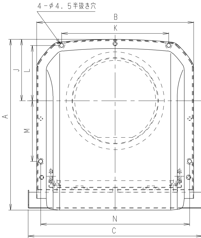
■ 寸法表
