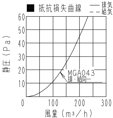
■ 抵抗損失曲線
