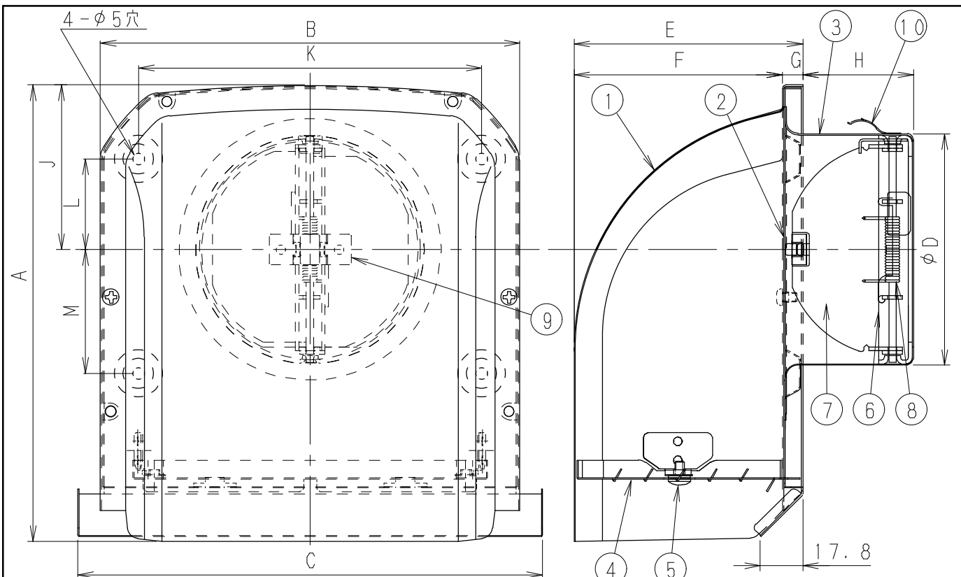
■ 寸法表
