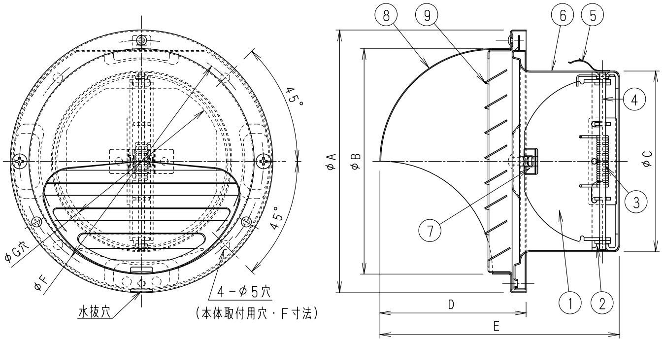
■寸法表
