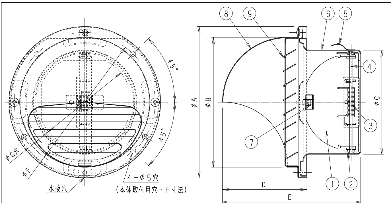
■寸法表
