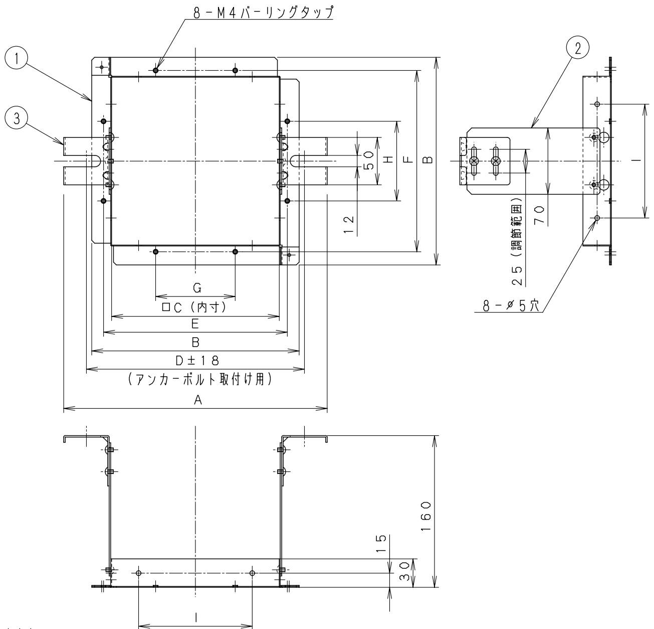
■寸法表
