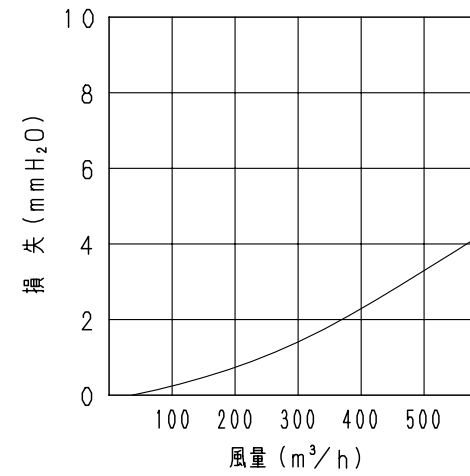
■ 抵抗損失曲線
