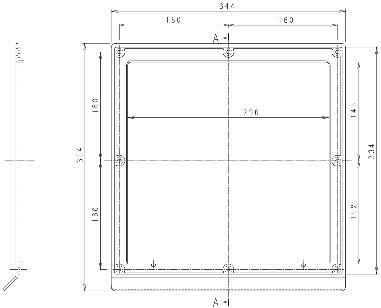
A-A SEC.
