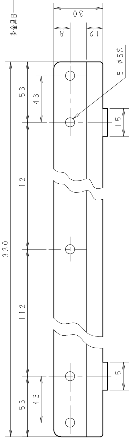
掛金具B
