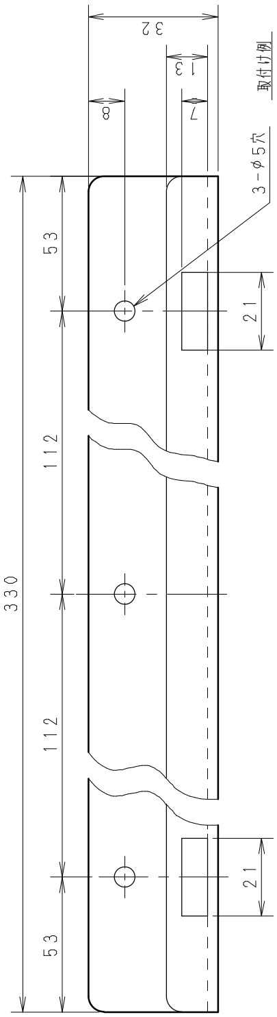
掛金具A
