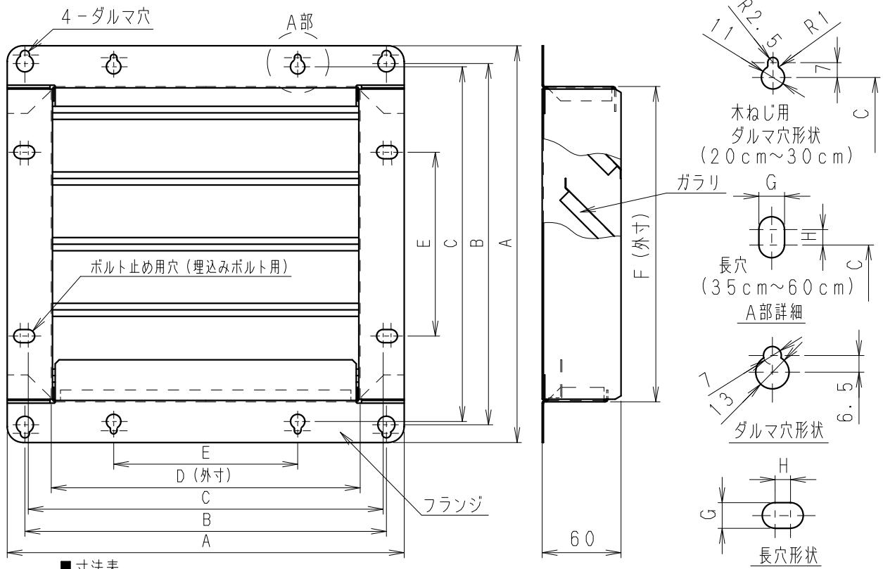
■寸法表
