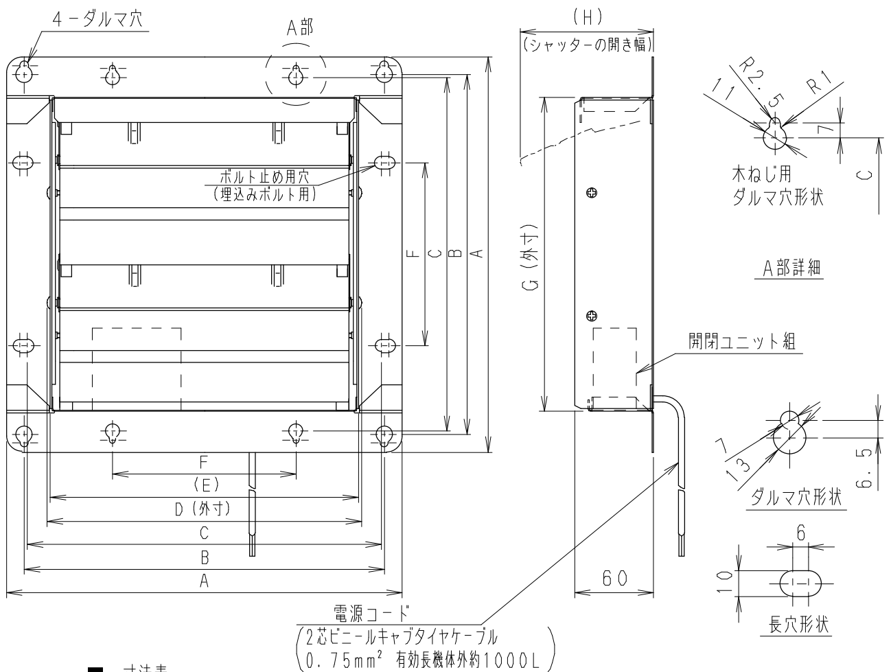
■ 寸法表
