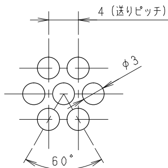
パンチング形状 (2:1)
