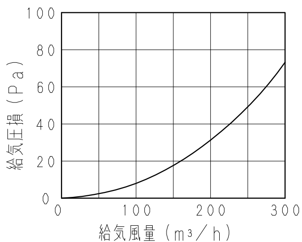
■抵抗損失曲線（給気圧損）
