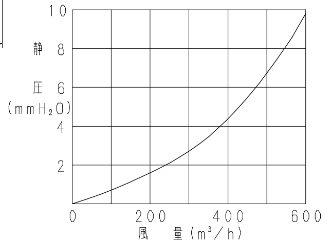
■ 抵抗損失曲線
