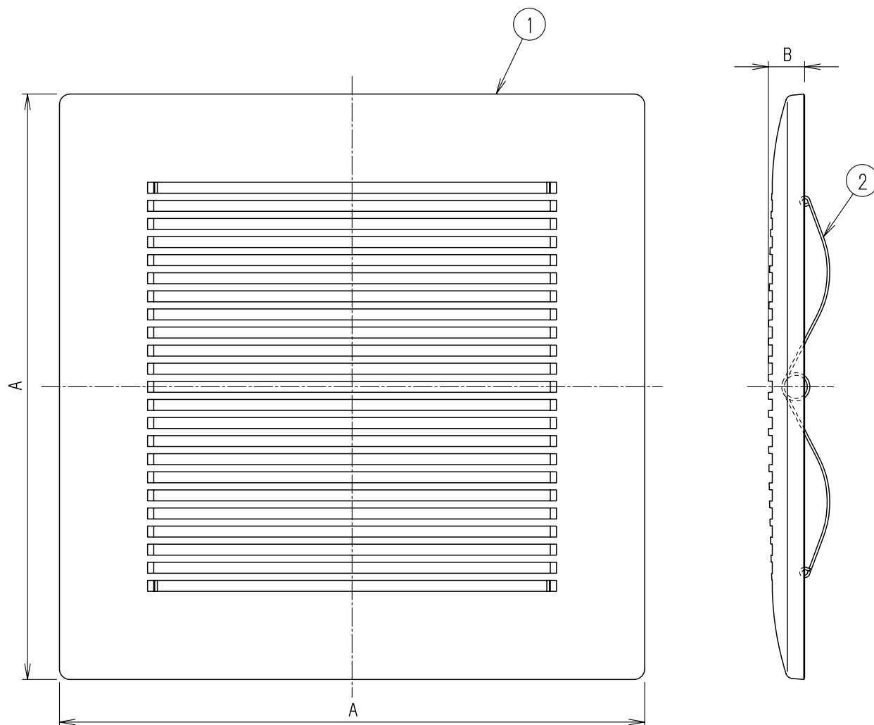
■ルーバー寸法表 (単位: mm)
