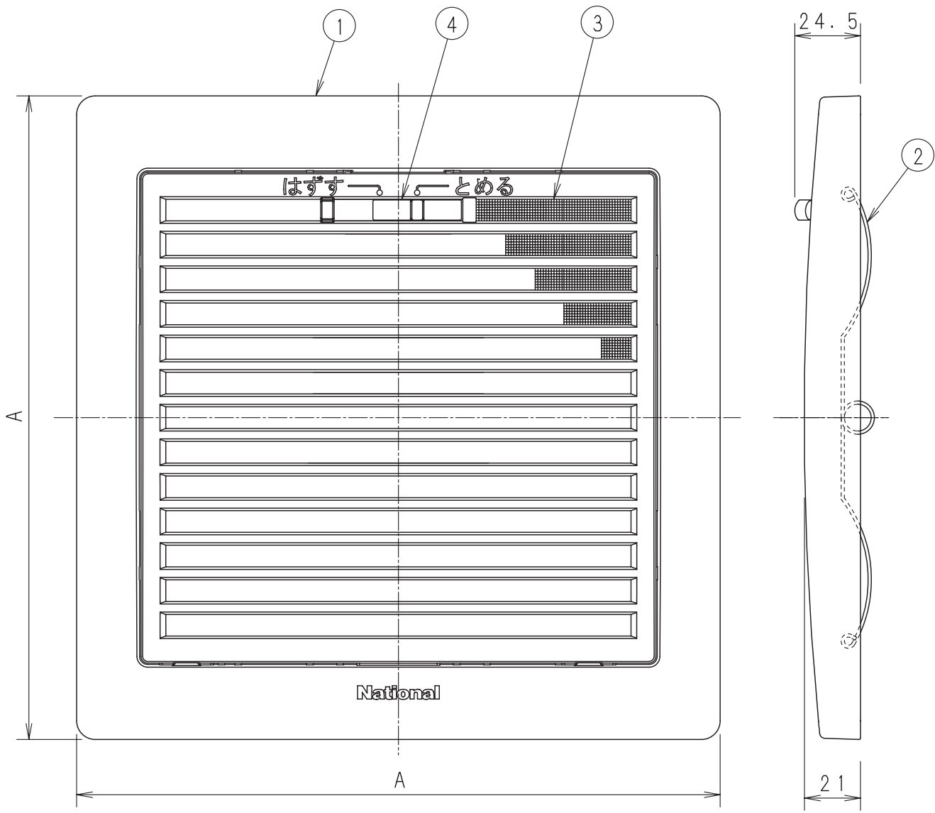
■ルーバー寸法表 (単位：mm)
