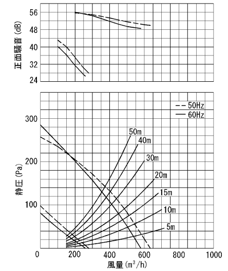
■特性表 (適用製品と本体カバー (DV-X23RV (K)) を組み合わせた場合の特性値です。)
