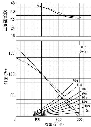
■静圧・風量・騒音特性 (DVF-XT18 φ150) 抵抗曲線はスパイラル管φ150の場合
