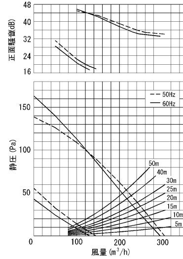
■静圧・風量・騒音特性 (DVF-XT18DA φ150) 抵抗曲線はスパイラル管φ150の場合
