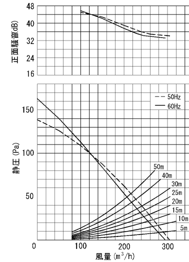
■静圧・風量・騒音特性 (DVF-XT18Y φ150) 抵抗曲線はスパイラル管φ150の場合
