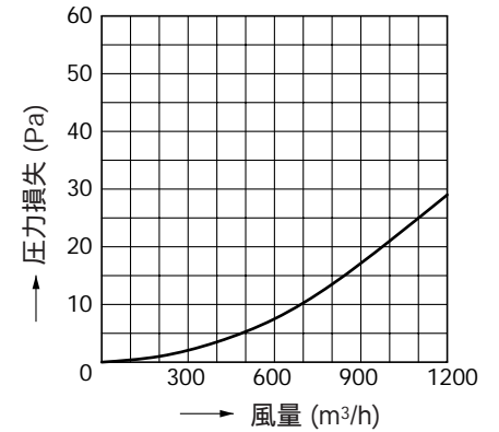
圧力損失曲線 使用パイプ 鋼板スパイラルダクトφ300 (内径φ300) 圧力損失係数 = 2.08
