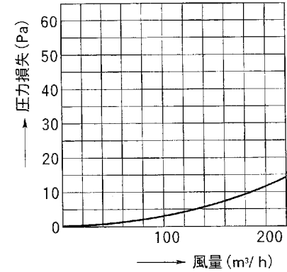
●DV-14JA 圧力損失曲線 (直線1m当り)
