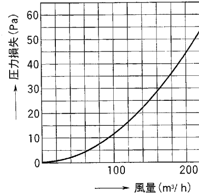
●DV-07JA 圧力損失曲線 (直線1m当り)
