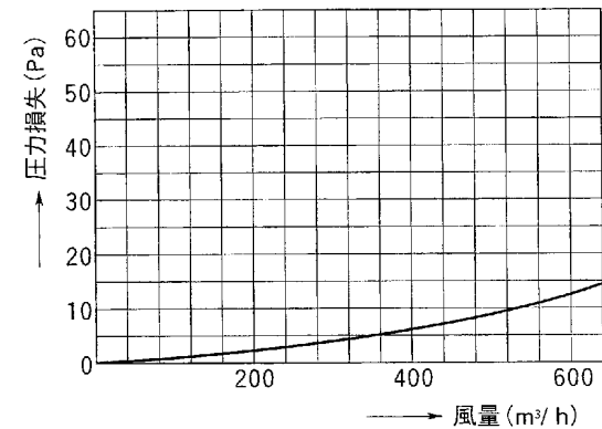
●DV-20JA 圧力損失曲線 (直線1m当り)
