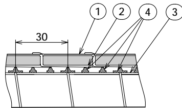
断面詳細図
