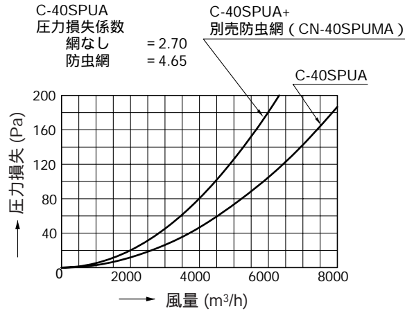
圧力損失曲線：給気
