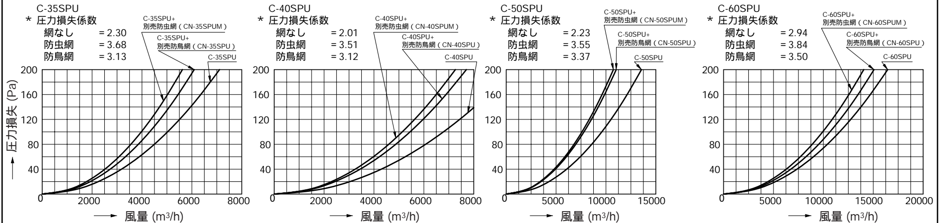
圧力損失曲線：給気
