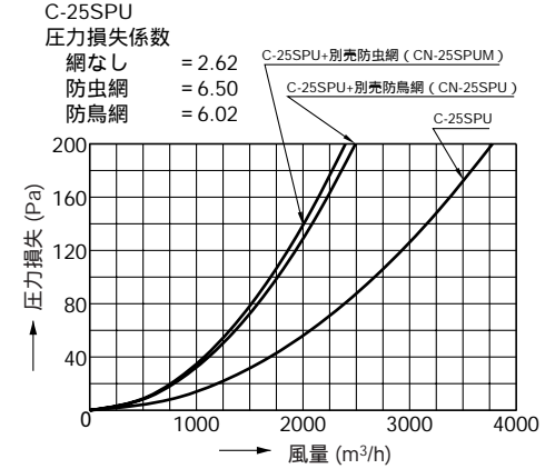
圧力損失曲線：給気
