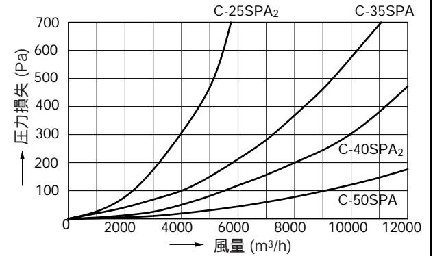
圧力損失曲線：給気
