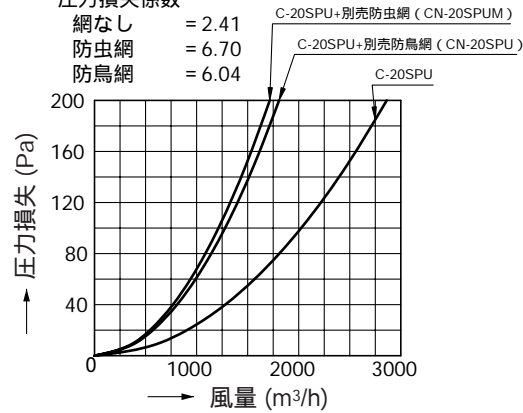
圧力損失曲線：給気
