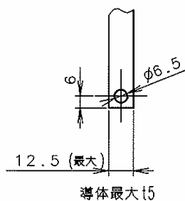
導体加工図
