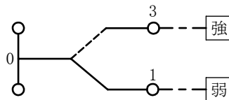
内部回路図
