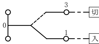
内部回路図
