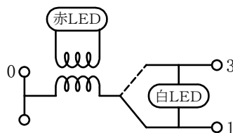
内部回路図
