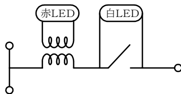
内部回路図
