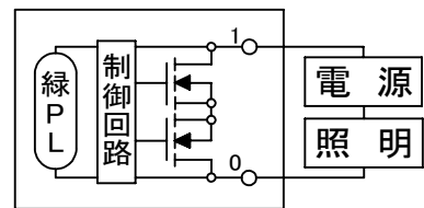
内部回路図
