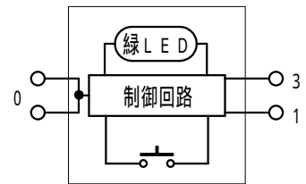
内部回路図
