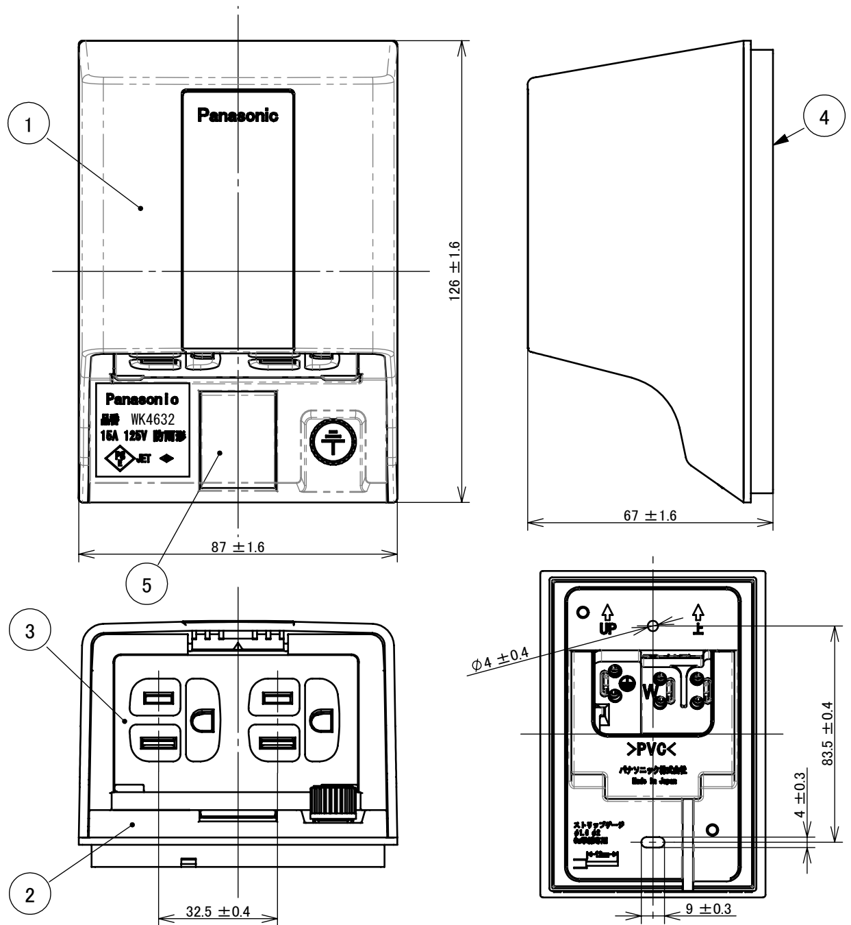
裏面 取付寸法(1:2)
