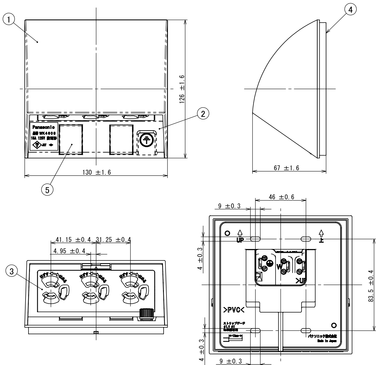
裏面 取付寸法(1:2)
