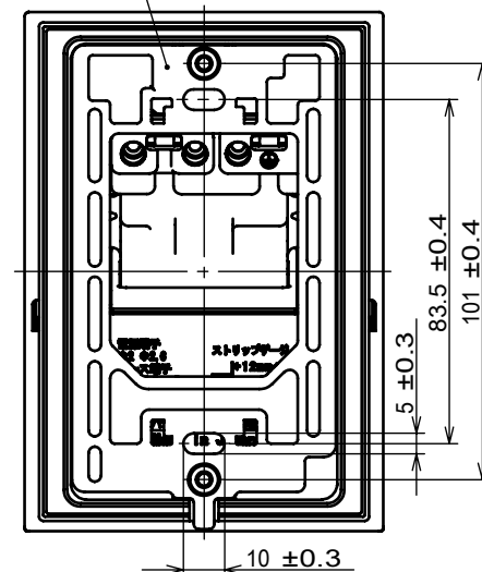
裏面 取付寸法
