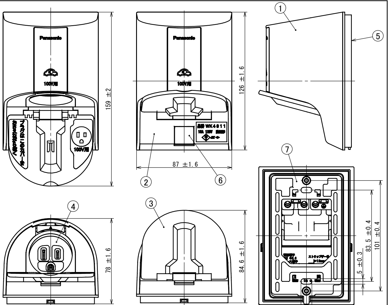
コンセントカバーを開いた状態
