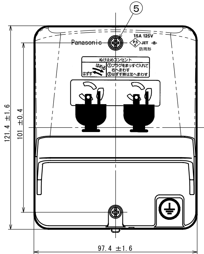
WK9905K 防水ブッシング使用時の 取付枠突起部までの寸法
