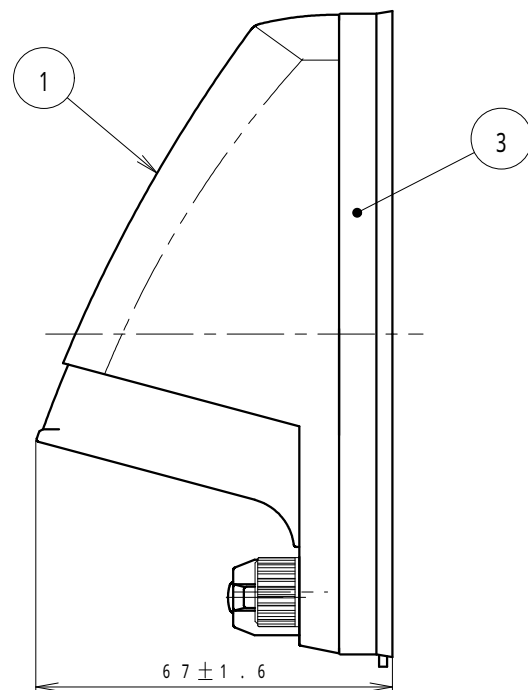
WK9905K 防水ブッシング使用時の 取付枠突起までの寸法
