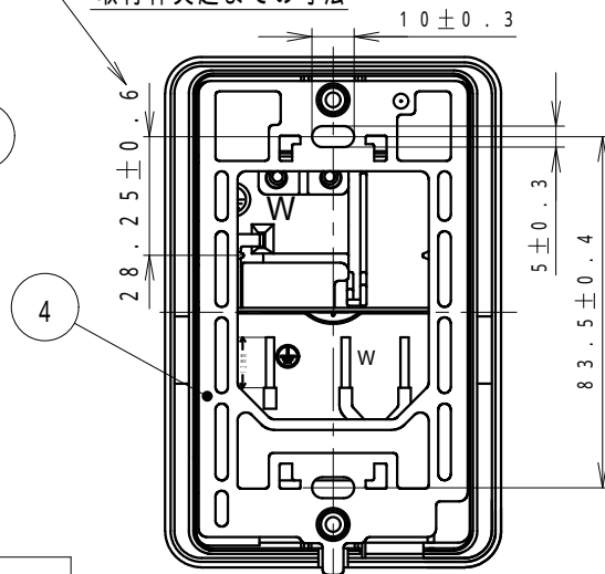
裏面取付寸法 (1:2)
