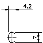
取付穴寸法
