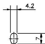
取付穴寸法
