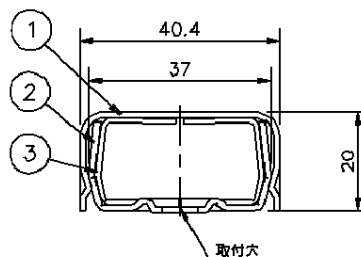
A-A断面
