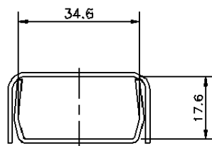
B-B断面
