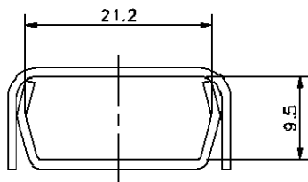
B-B断面
