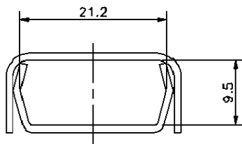
B-B断面
