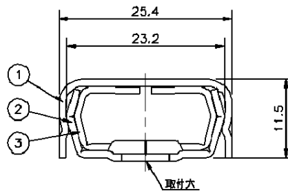
A-A断面
