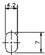
取付穴寸法
