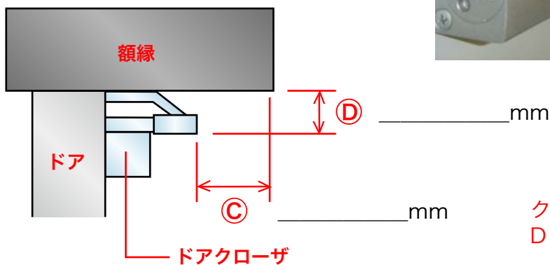
クローザ部分 側面図
