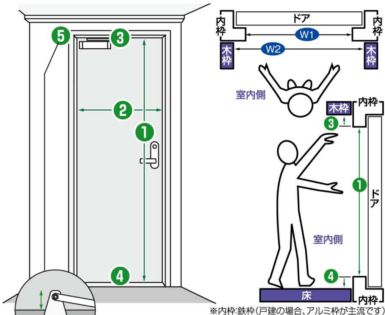
ドアクローザー 飛び出し
