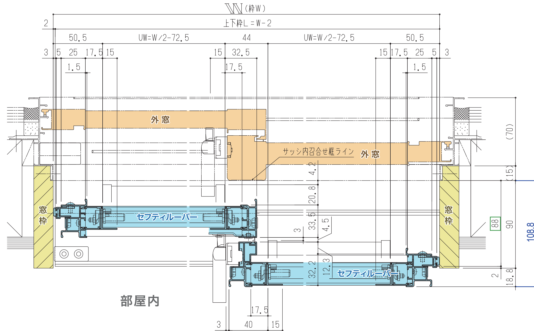
横断面 (2枚建て) テラスサイズ納まり図
