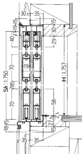
縦断面図 ③-E
