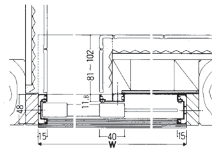
横断面図 ②-D
