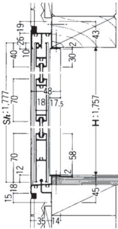
縦断面図 ①-A
