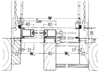
横断面図 ①-B
