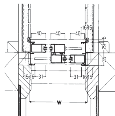
横断面図 ③-F
