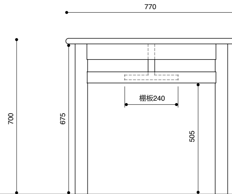
【側面】
