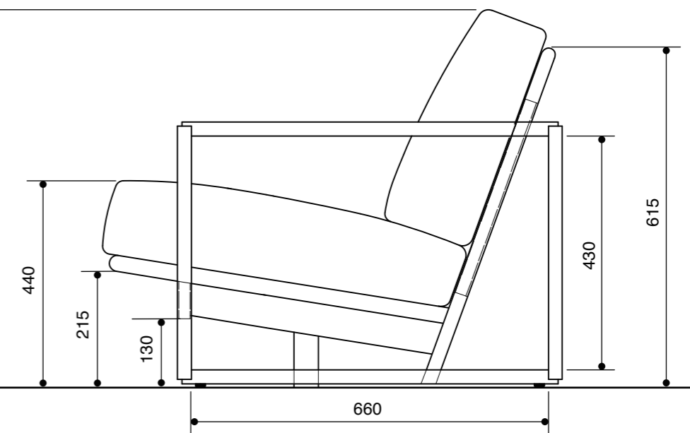
【側面】
