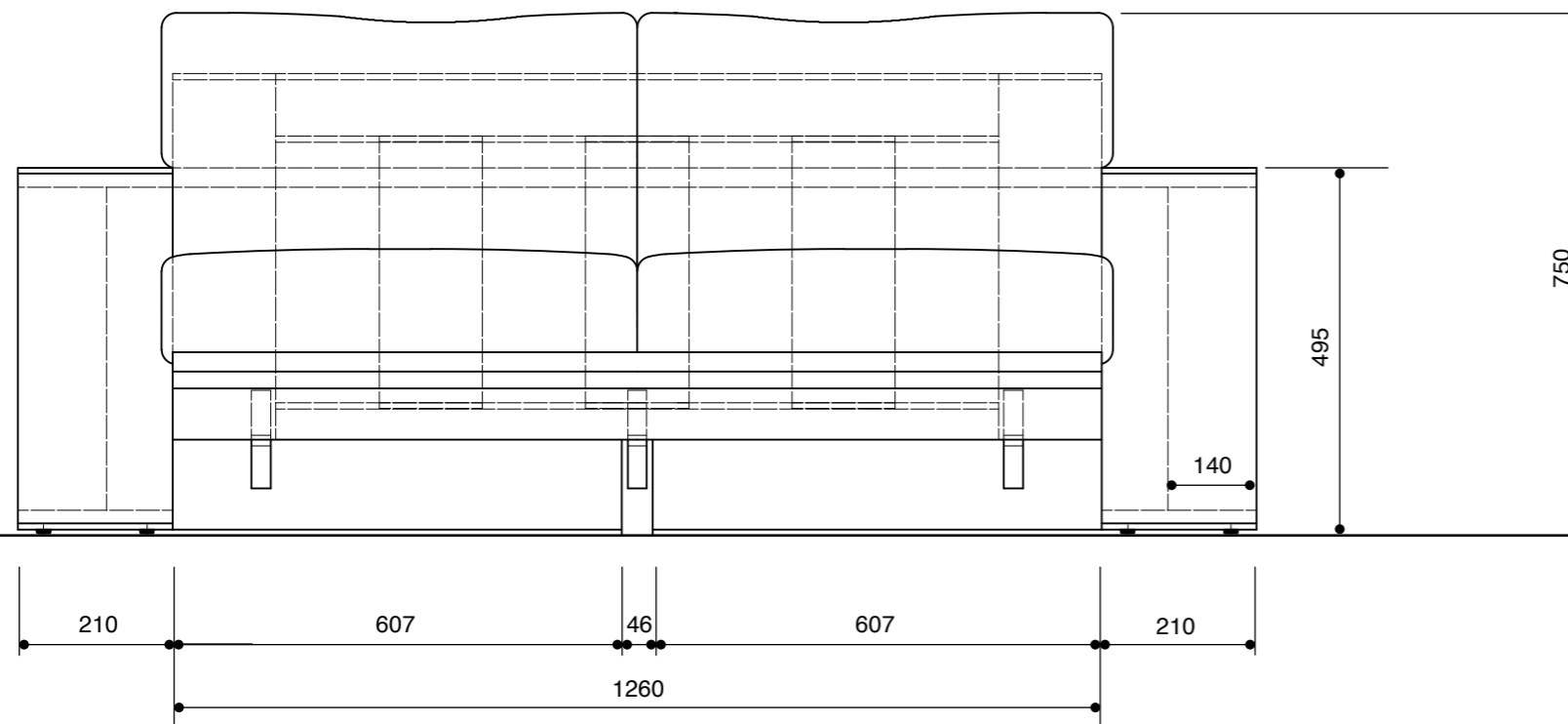
【正面】
