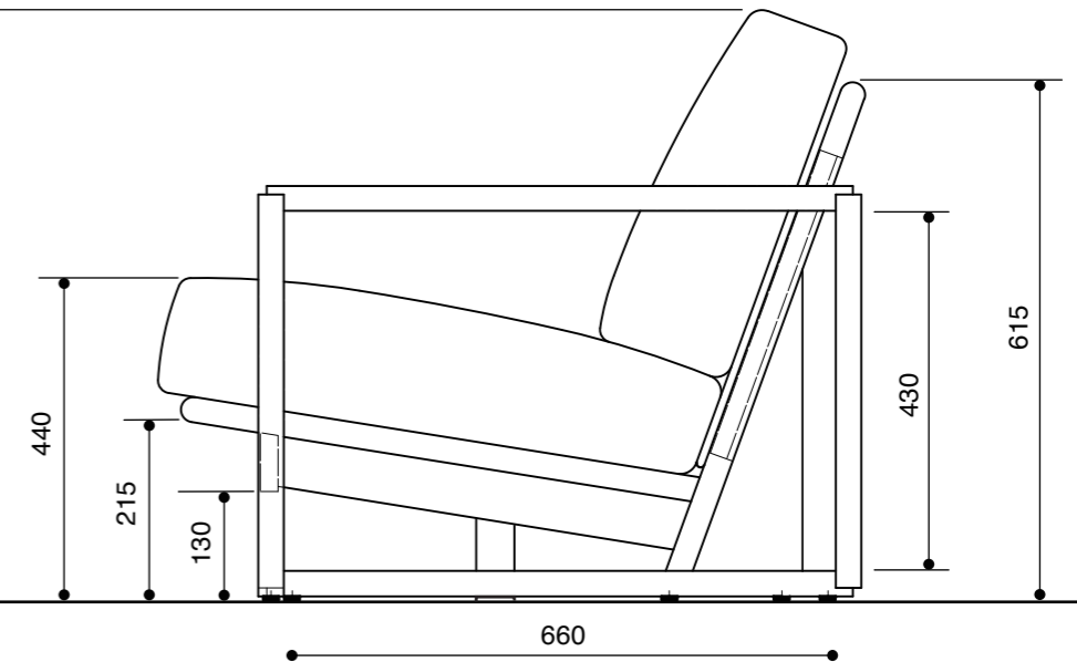
【側面】
