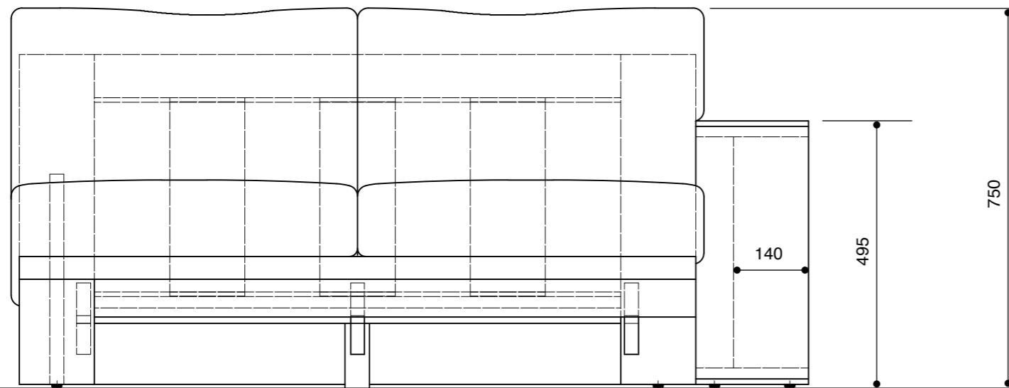
【正面】
