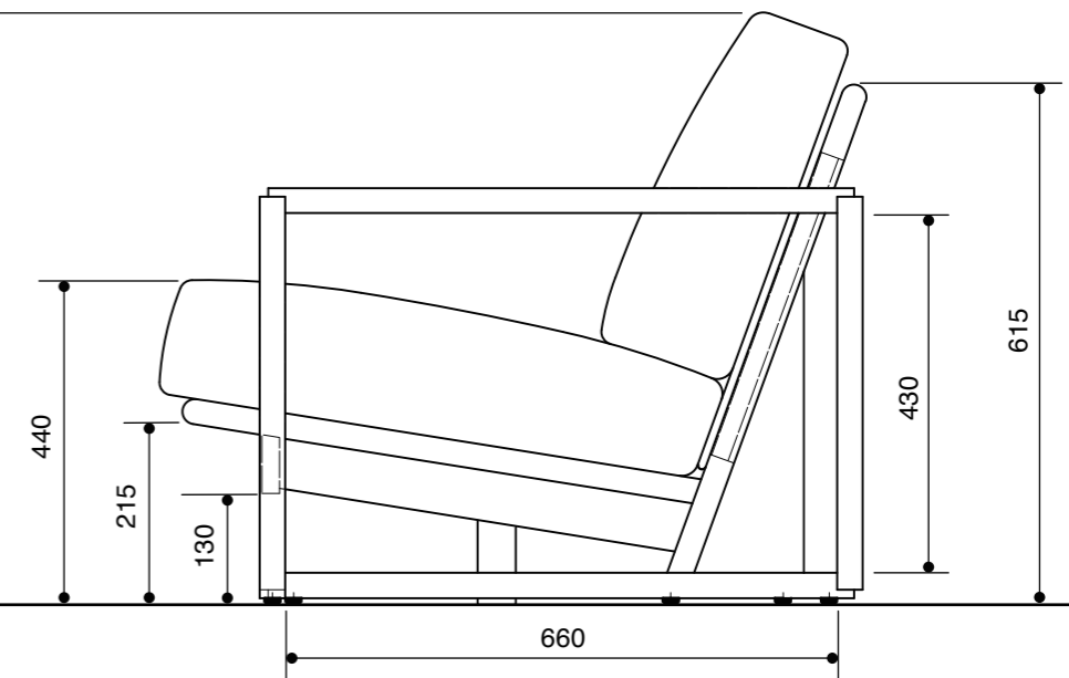
【側面】
